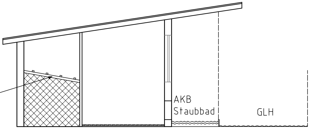
Variante 2: mit Kotgrube
