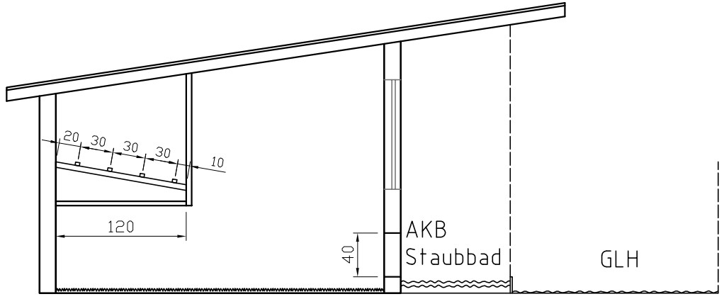
Variante 1: mit Kotbrett
